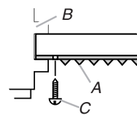
A. Cortina izquierda B. Canal de la ventana C. Tornillo de cabeza redonda #10 x \frac{3}{4} "
